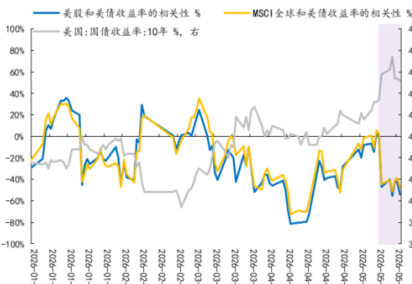
图表5：最近一周权益市场与美债之间的相关性相较之前开始出现逆转
